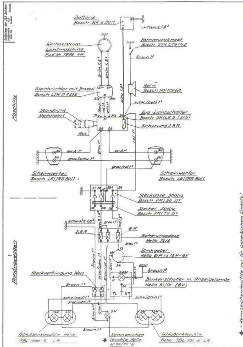
Schaltplan 6-Volt-Anlage an den Holder Einachsschleppern EF 9 – EB 9 – ED 10 – ED II – EB II – BED II – E 11 mit Holder Einachs-Anhängewagen Type 155
