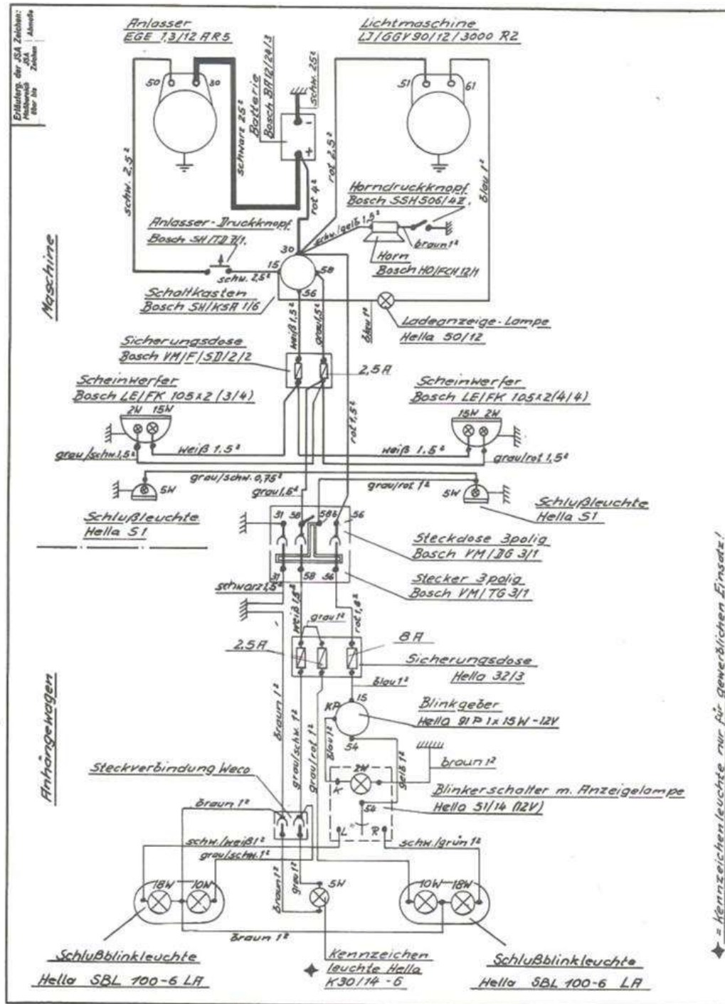
Schaltplan 12-Volt-Anlage am Holder Einachsschlepper E 12 mit Holder Einachs-Anhängewagen Type 155
